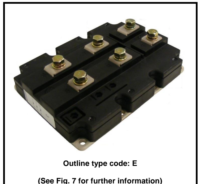
Fig. 2 Package
