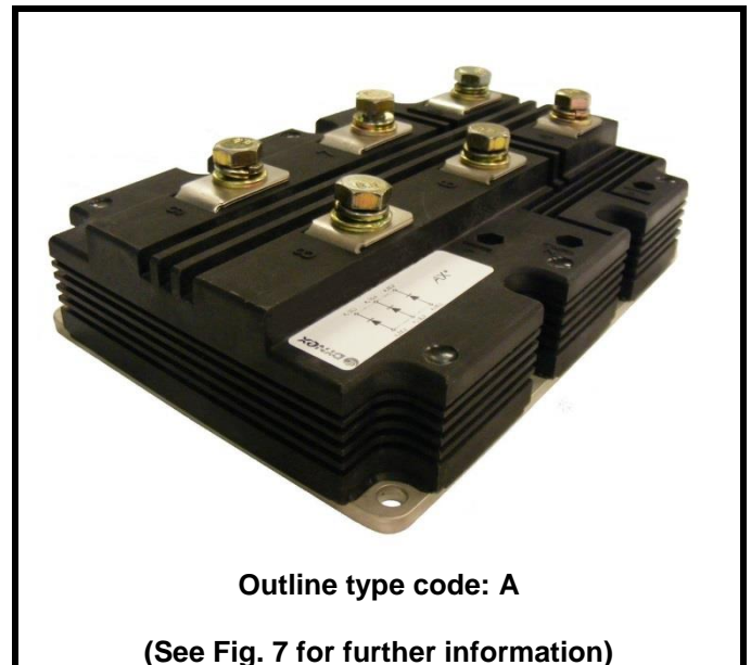
Fig. 2 Package
