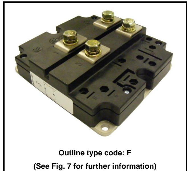
Fig. 2 Package
