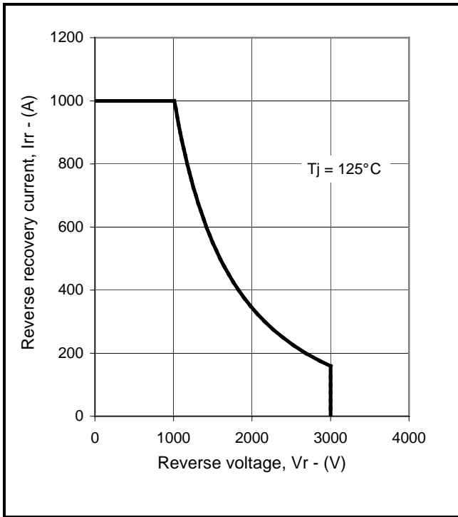
Fig.7 Diode RBSOA
